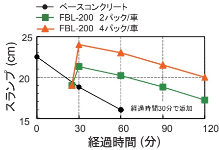
図1 スランプの経時変化
