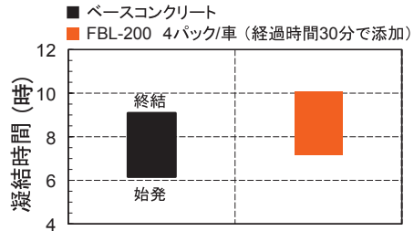
図4 凝結試験結果
