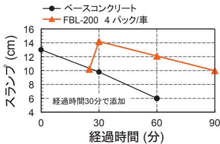
図3 スランプの経時変化
